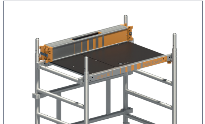
2. Bordbretteinheit 12 einseitig an den Holmen der Standleiter anlegen
